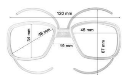
AGGIUNTIVO OTTICO GEKO-JR KIT OPTIK GEKO-JR
